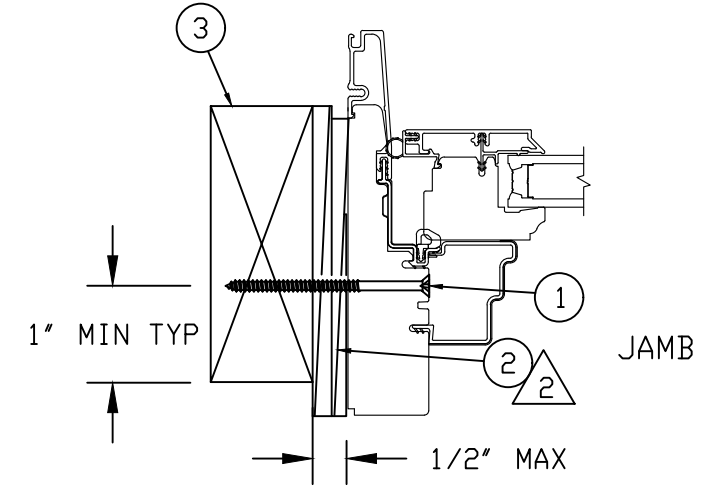
HEAD JAMB
